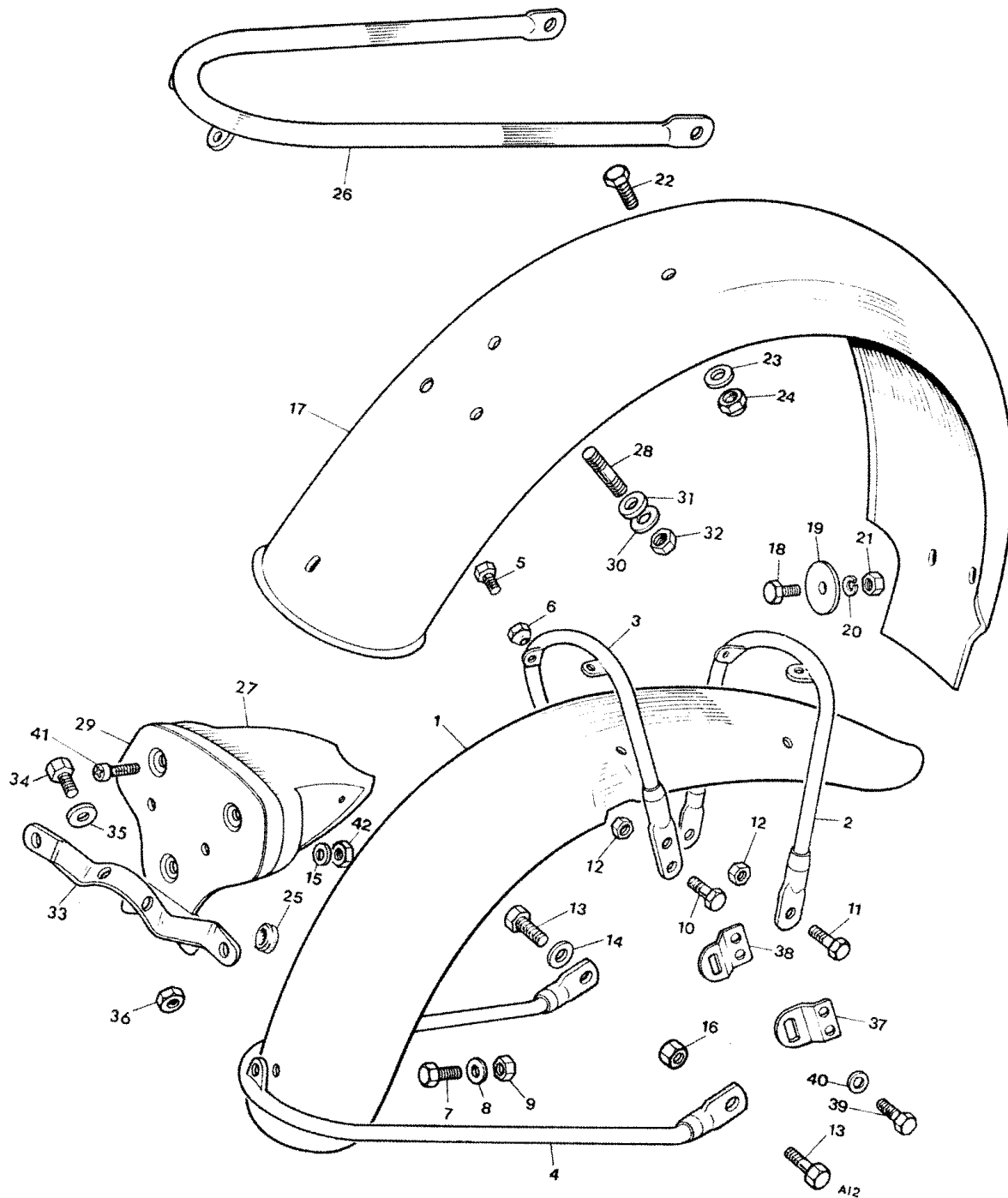
Fig. 12. FENDERS
