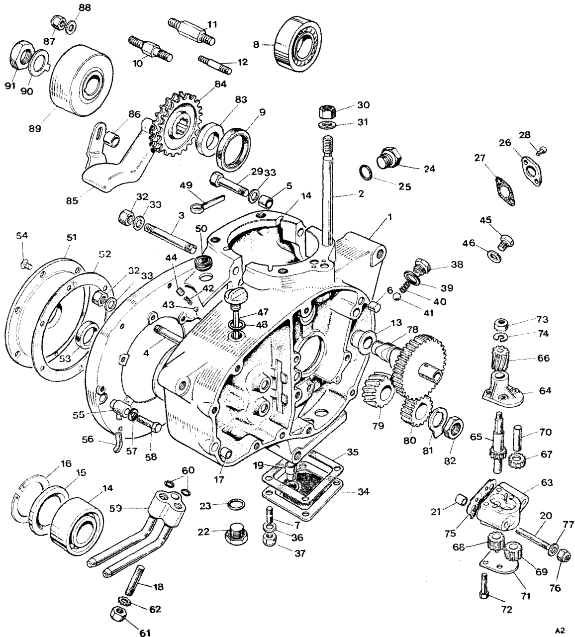
Fig. 2. CRANKCASE
