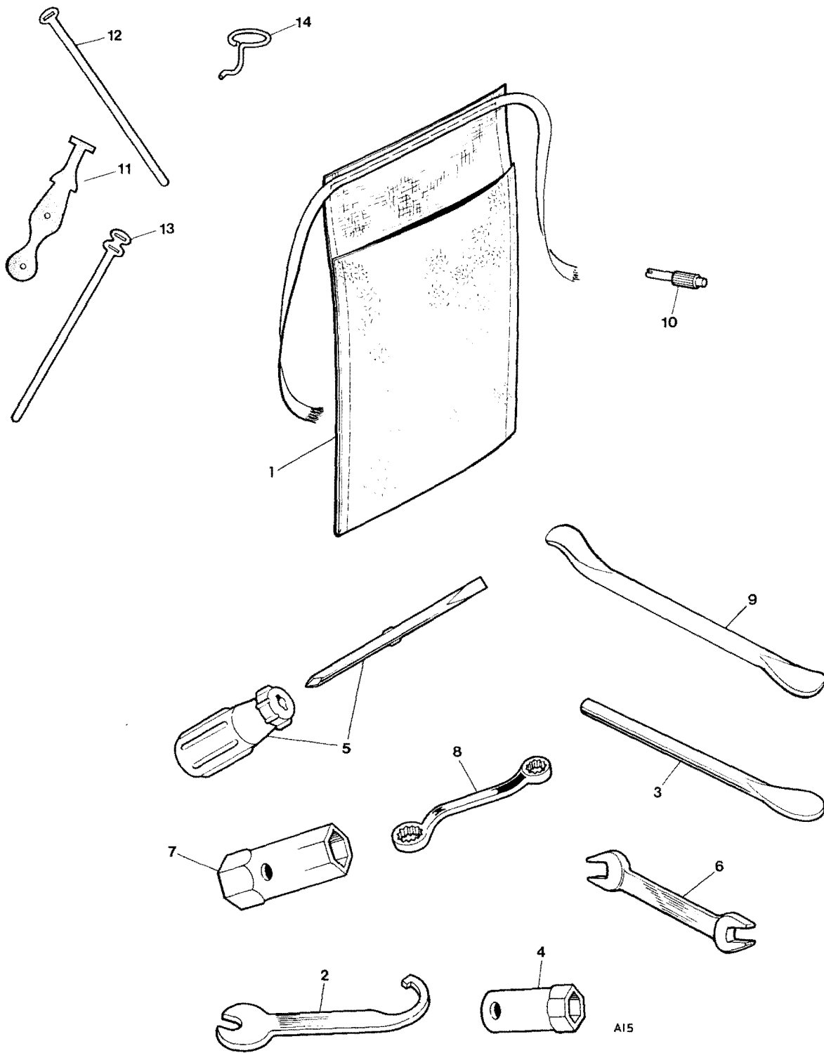
Fig. 17. TOOL KIT
