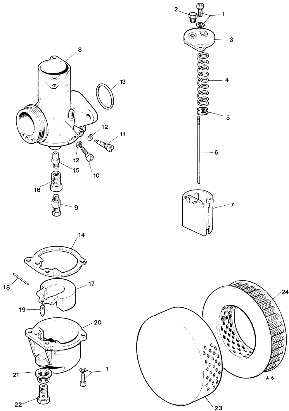
Fig. 18. CARBURETOR
