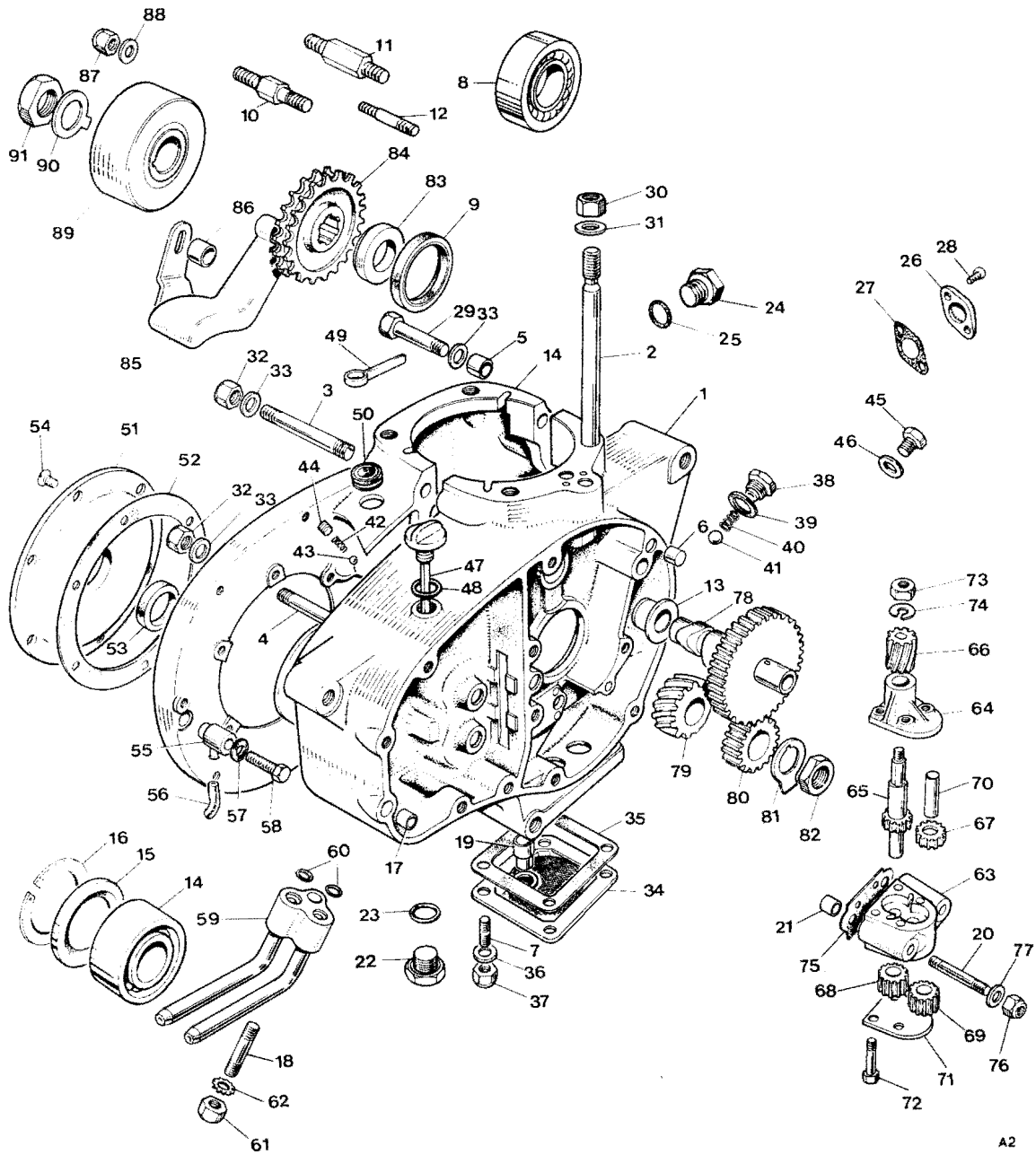
Fig. 2. CRANKCASE
