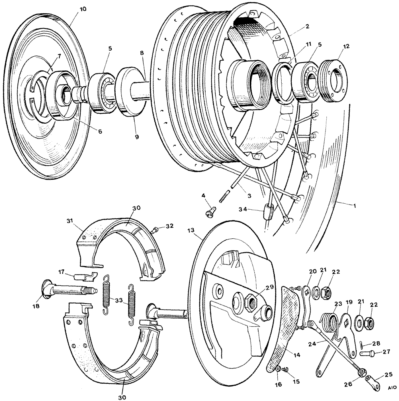
Fig. 10. FRONTWHEEL
